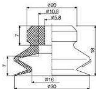
Durchmesser Sauger \phi 30
