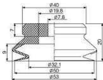
Durchmesser Sauger \phi 50
