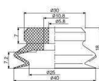
Durchmesser Sauger \phi 40
