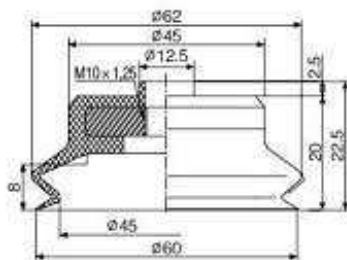
Durchmesser Sauger \phi 60
