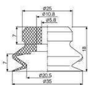
Durchmesser Sauger \phi 35
